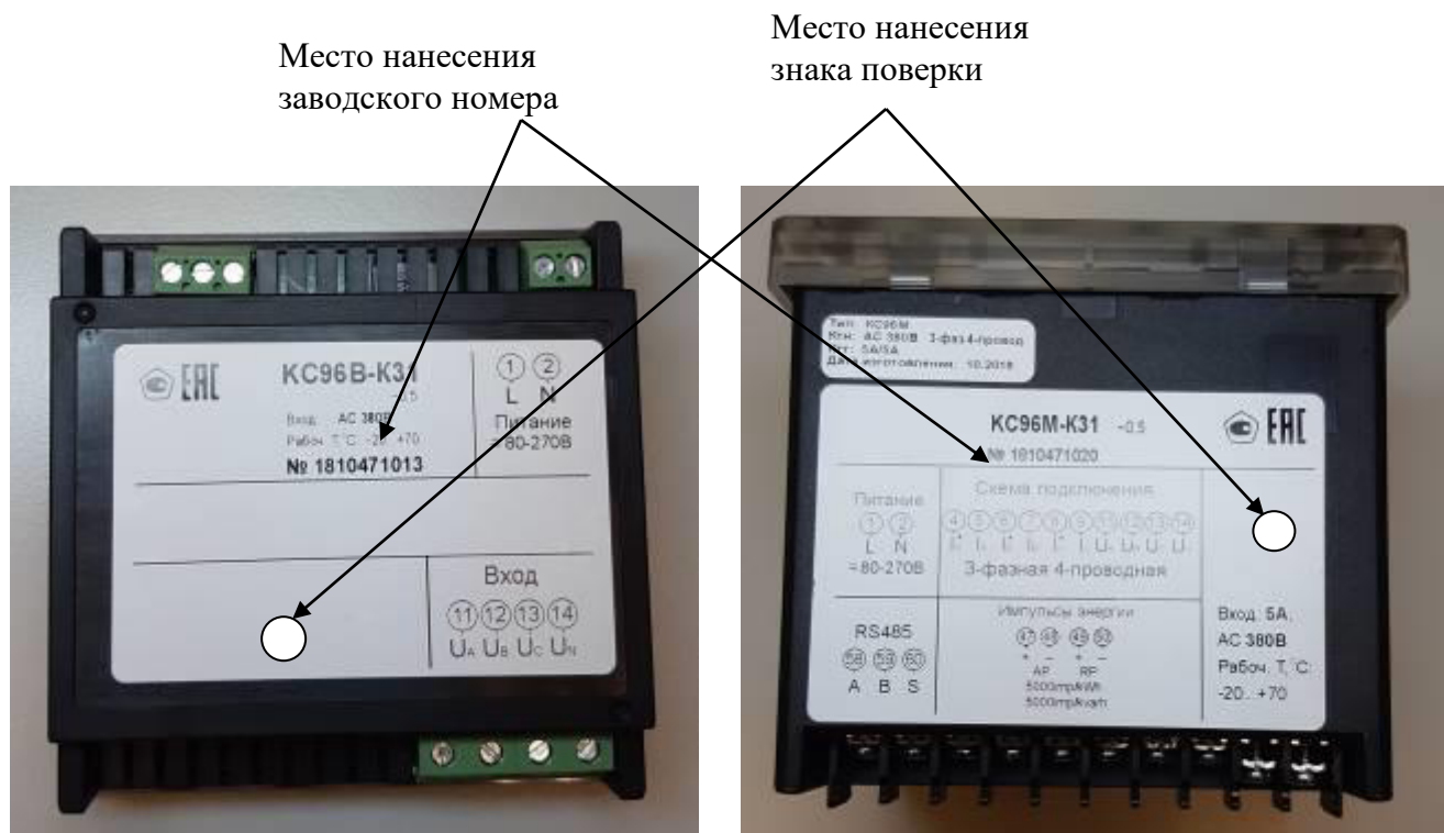
Рисунок 14 – Общий вид приборов KC96B. (трехфазная модификация). Вид сзади
